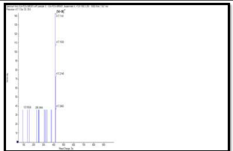
Diadizein-C-hexoside
