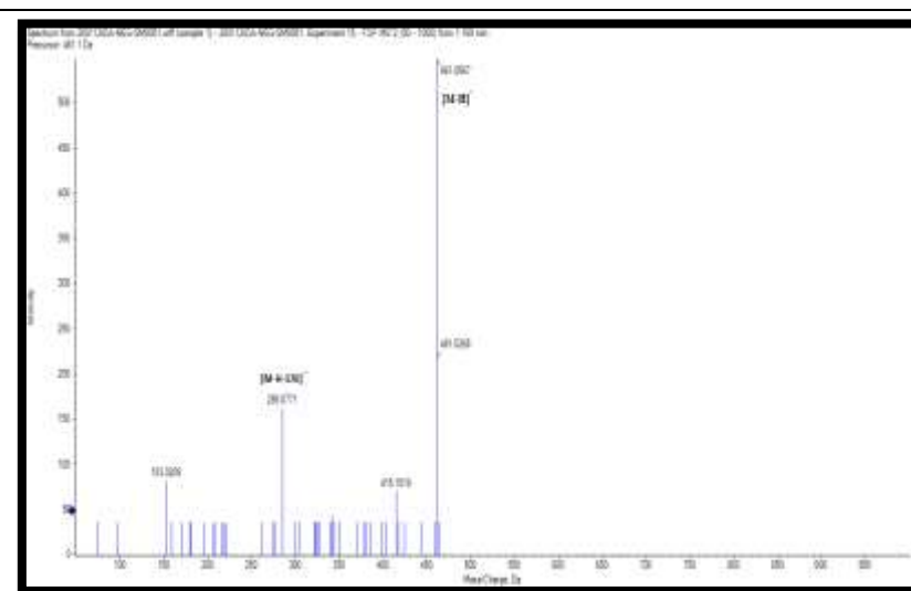
Kaempferol-O-hexouronide
