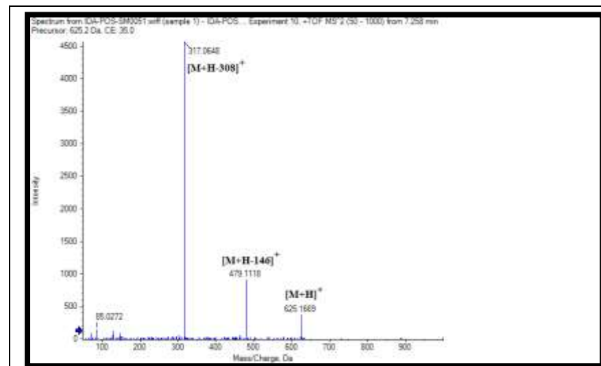
Isorhamnetin-3-O-rutinoside
